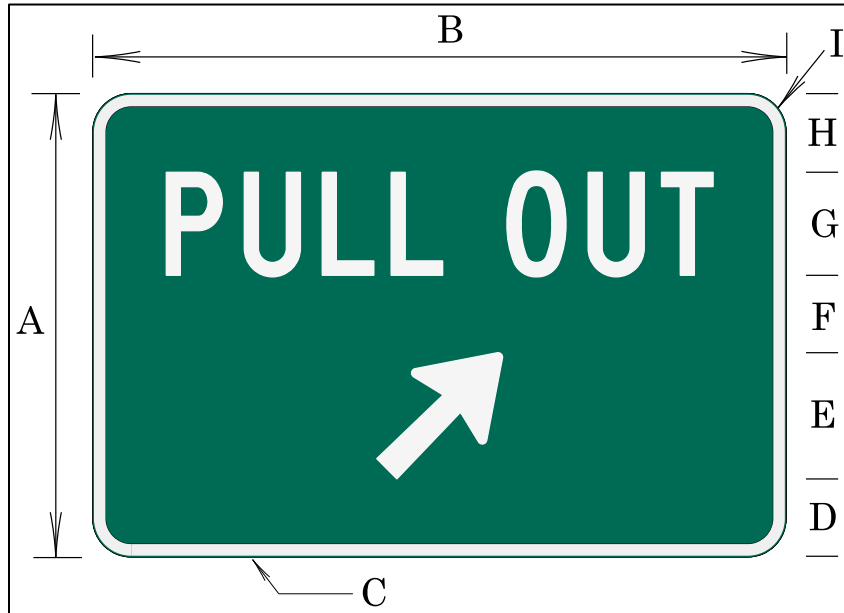
Figure 102: Sign OD12-1 (PULL OUT) Detail
