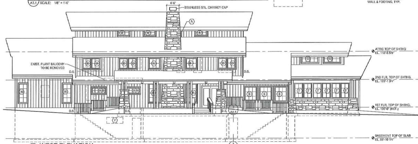
4 WEST ELEVATION A3.1 SCALE: 1/8" = 1'-0"
