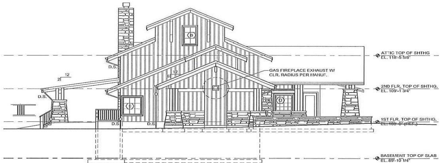
1 SOUTH ELEVATION A3.1 SCALE: 1/8" = 1'-0"
