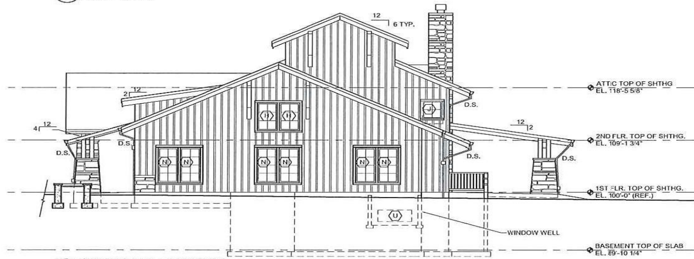
3 NORTH ELEVATION A3.1 SCALE: 1/8" = 1'-0"
